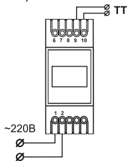
Схема подключения
