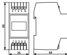
Габаритные размеры
