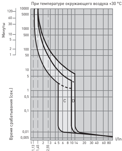
Рис. 1 - Время-токовые характеристики
