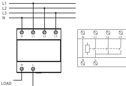
Рис. 6 - Схема подключения
