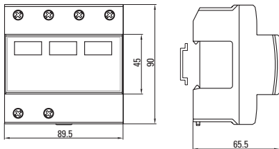
Рис. 7 - Габаритные и установочные размеры
