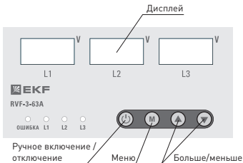
Рис. 4 - Дисплей и индикация
