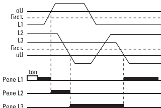
Рис. 2 - Диаграммы работы реле без возврата к приоритетной фазе
