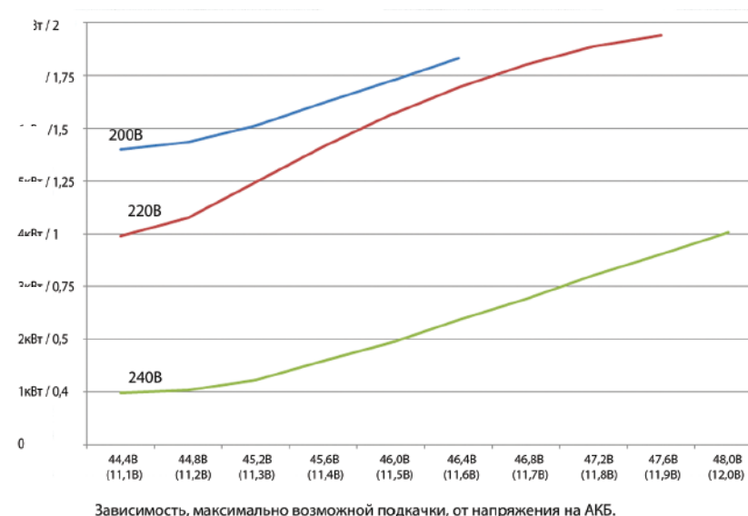
Рисунок 7. Зависимость максимально возможной подкачки от напряжения на АКБ и напряжения в сети.
